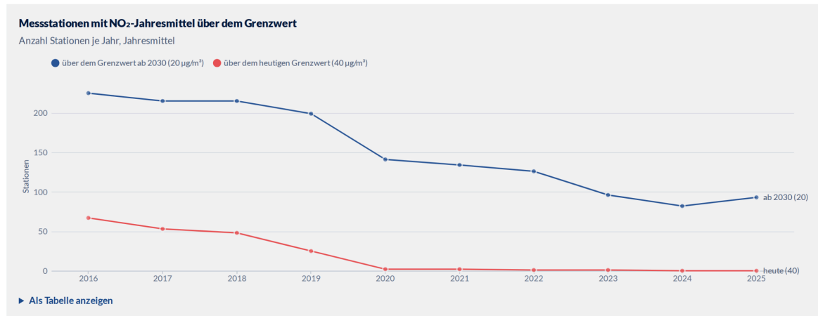
Abb. 1: Messstationen mit NO 2 -Jahresmittel über dem Grenzwert. Rot: heutiger Grenzwert (40 µg/m 3 ), 2025 keine Station mehr. Blau: Grenzwert ab 2030 (20 µg/m 3 ), 2025 noch 93 Stationen. Hinweis: Daten des Referenzangebots; maßgeblich ist die amtliche Auswertung des Umweltbundesamts [M1], [3].
